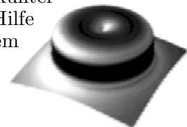
Abb. 5: „Hut“, erzeugt mit DPGraph
