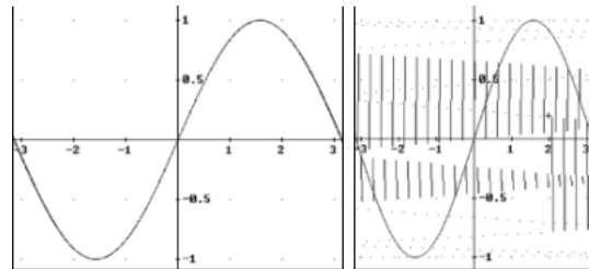
Abb. 12: Simulation von \sin(x) und \sin(ax) (mit a = ? ) mittels Derive, nur die Fenstergröße wurde variiert.
