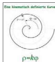
Abb. 2.11: Archimedische Spirale
